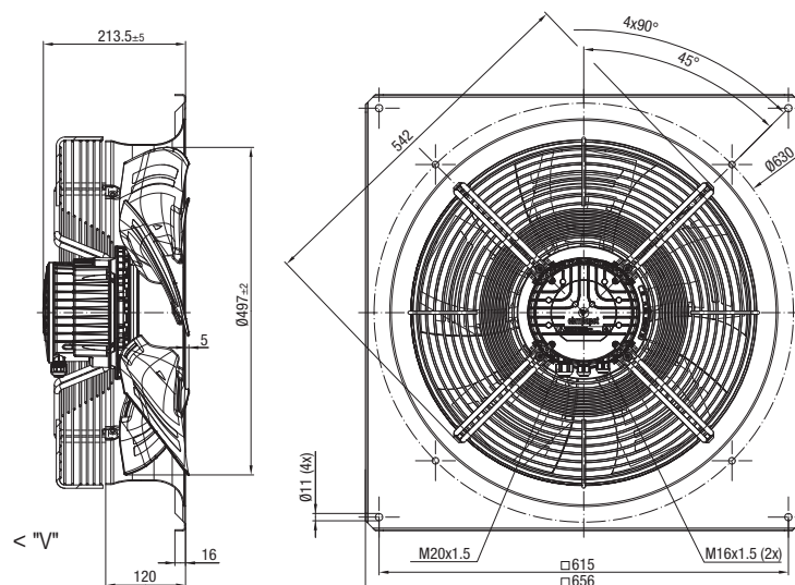
S3G 500-AA74-21 (с защитной решеткой для короткого диффузора, направление воздушного потока "V")
