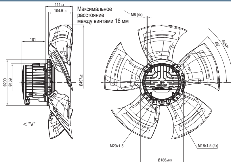
W3G 500-GA74-21 (с квадратным полнопропускным корпусом, направление воздушного потока "V")
