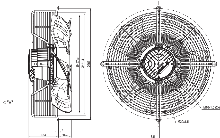
S3G 500-AA74-21 (с защитной решеткой для короткого диффузора, направление воздушного потока "V")
